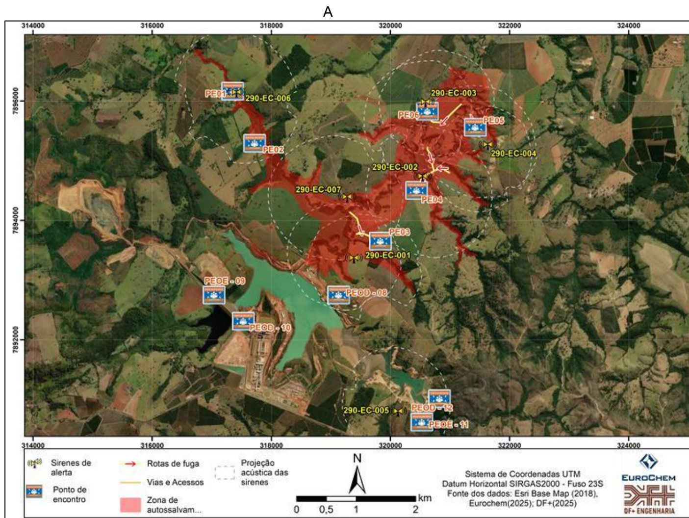
Figura 6.5 apresenta a localização das sirenes e suas respectivas projeções sonoras, pontos de encontro e rotas de fuga. .
