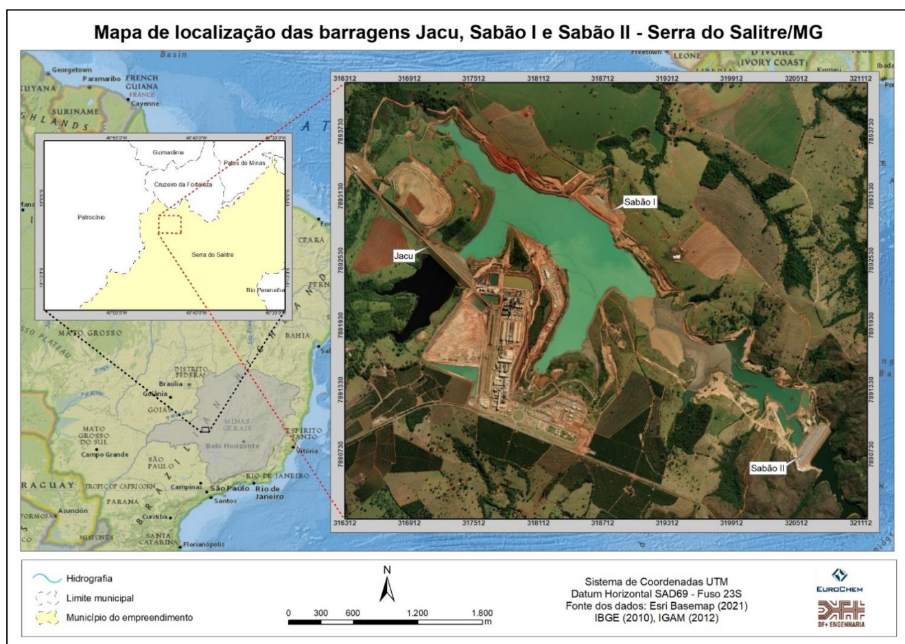
Figura 6.1 - Localização da Barragem Sabão II - CMISS - Complexo Minerio Industrial de Serra do Salitre.
