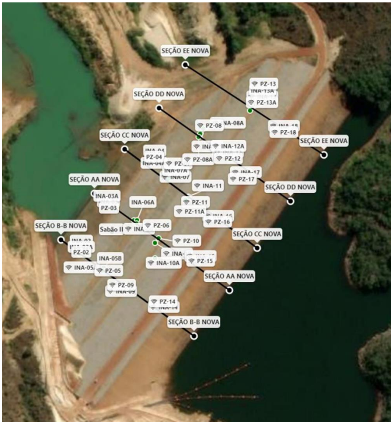
Figura 6.3 - Planta de localização do Sistema de Monitoramento da Barragem Sabão II – El. 982m
