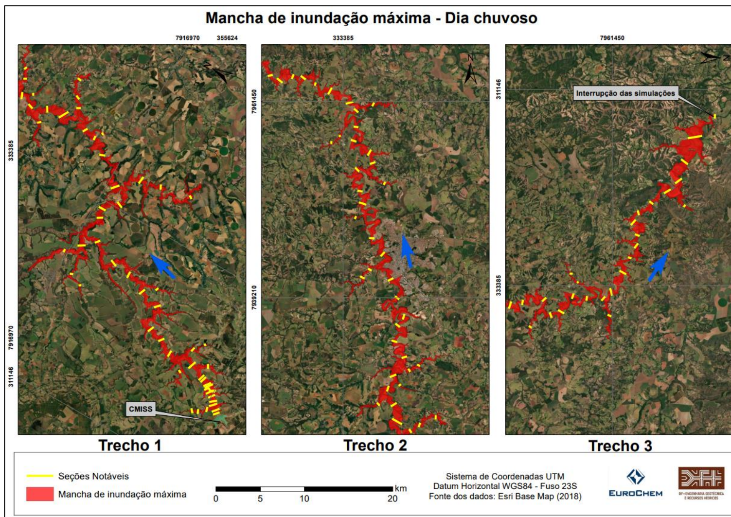
Figura 14.1 – Mancha de inundação máxima - Barragens Sabão I, Sabão II e Jacu.
